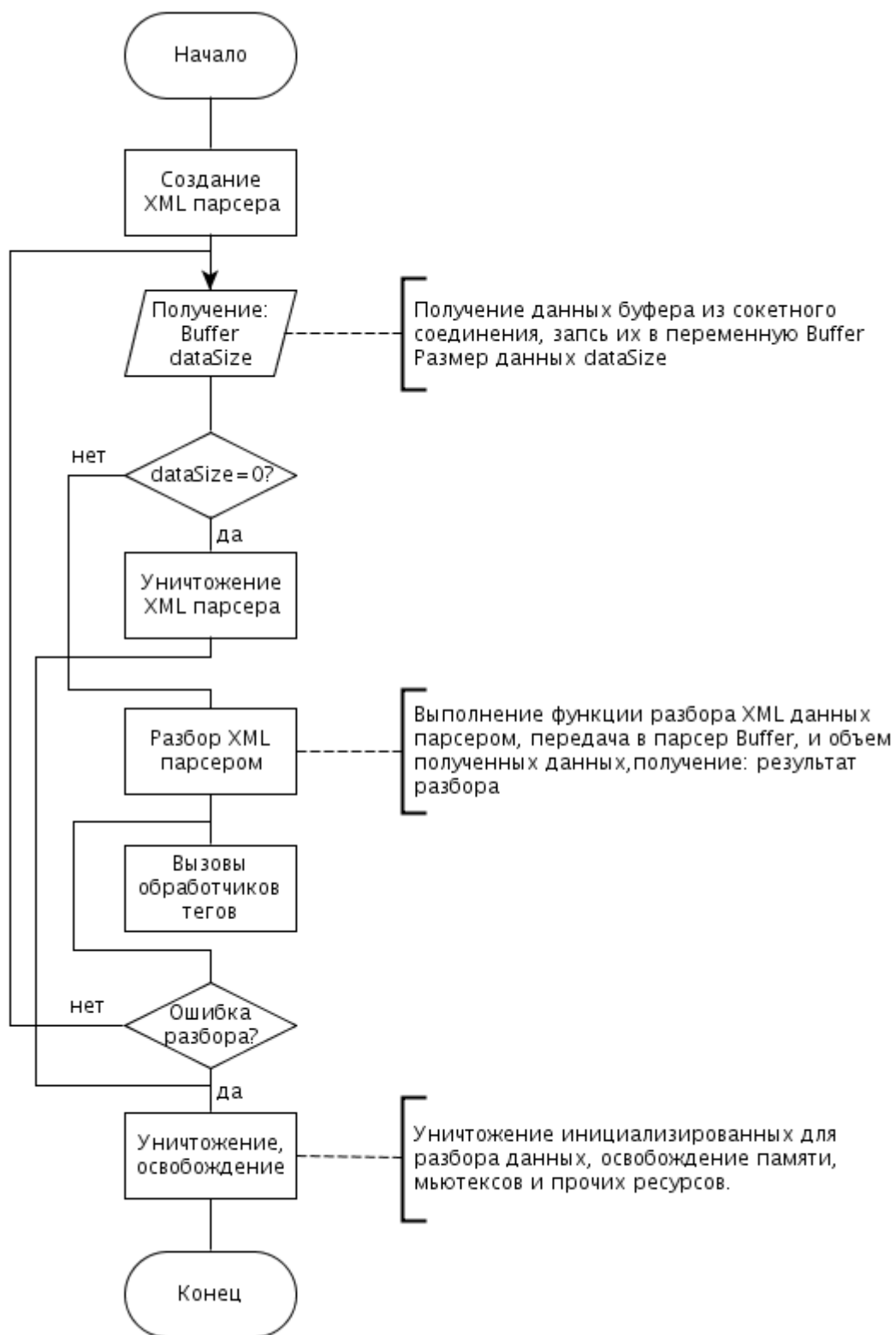
Рисунок 2.8 – Алгоритм разбора потокового XML
