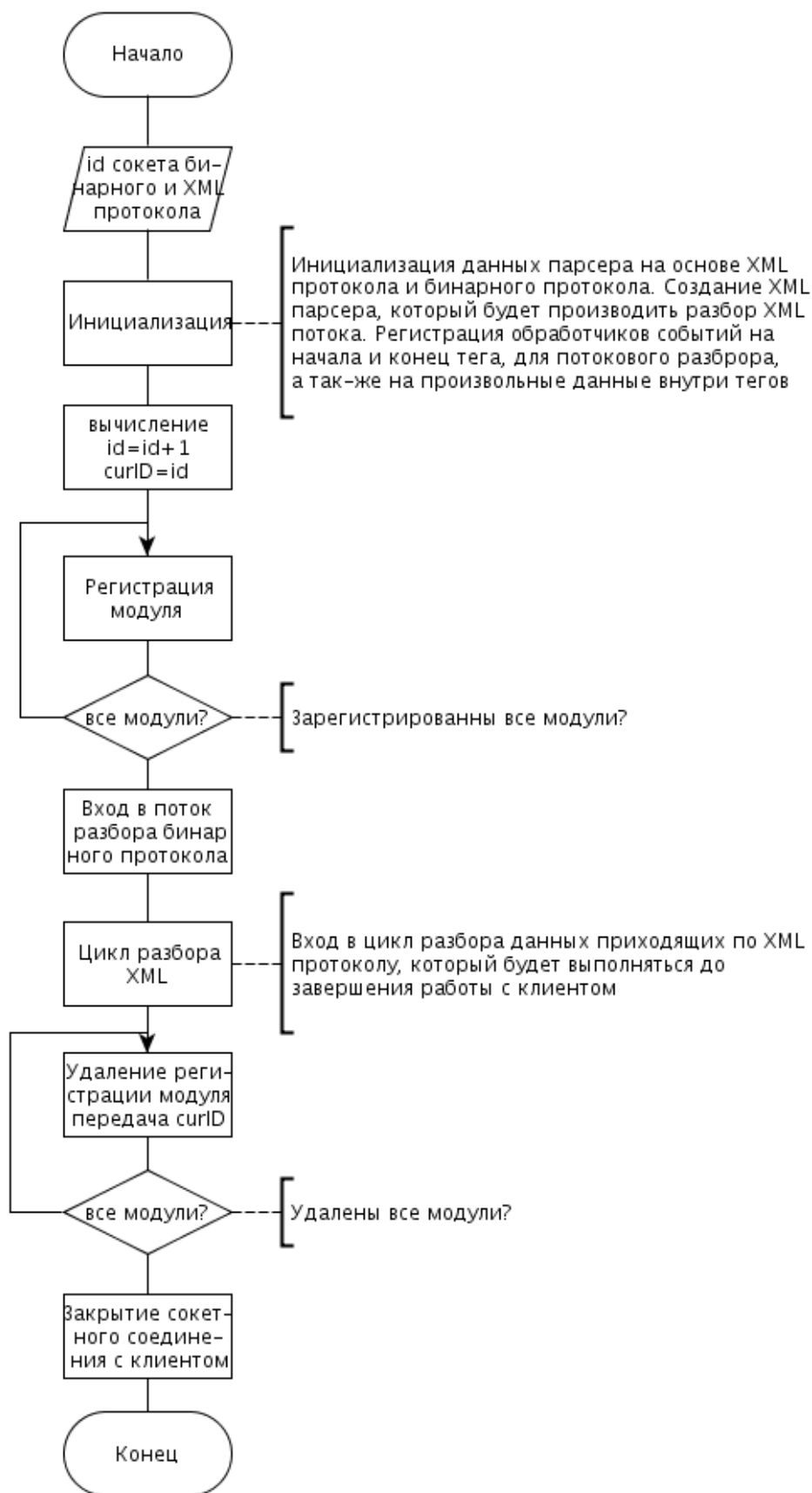
Рисунок 2.4 – Алгоритм цикла обработки клиента
