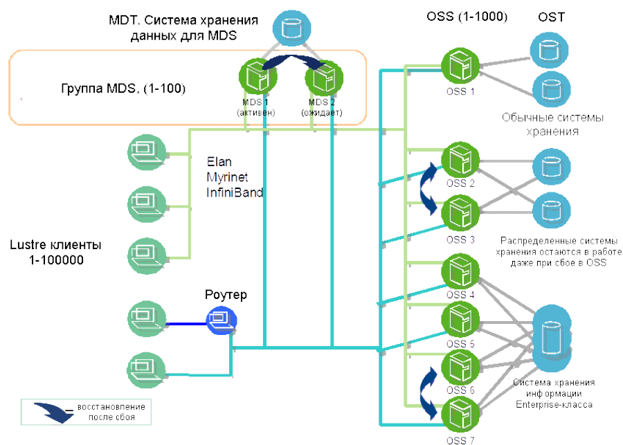
Рисунок 1 – Схема архитектуры системы Lustre
