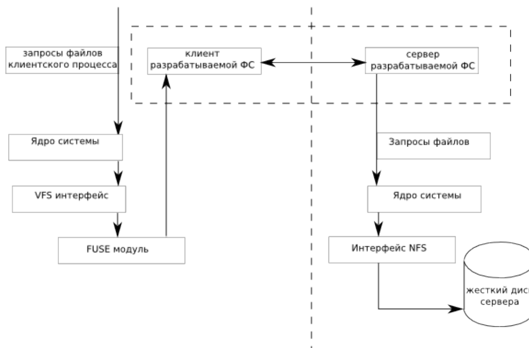
Рисунок 2.1 – Схема взаимодействие разрабатываемой программы с компонентами системы
