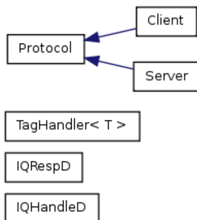
Рисунок 3.3 – Схема наследования классов бинарного протокола на основе XML.
