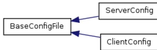
Рисунок 3.5 – Схема наследования классов чтения конфигурационного файла.
