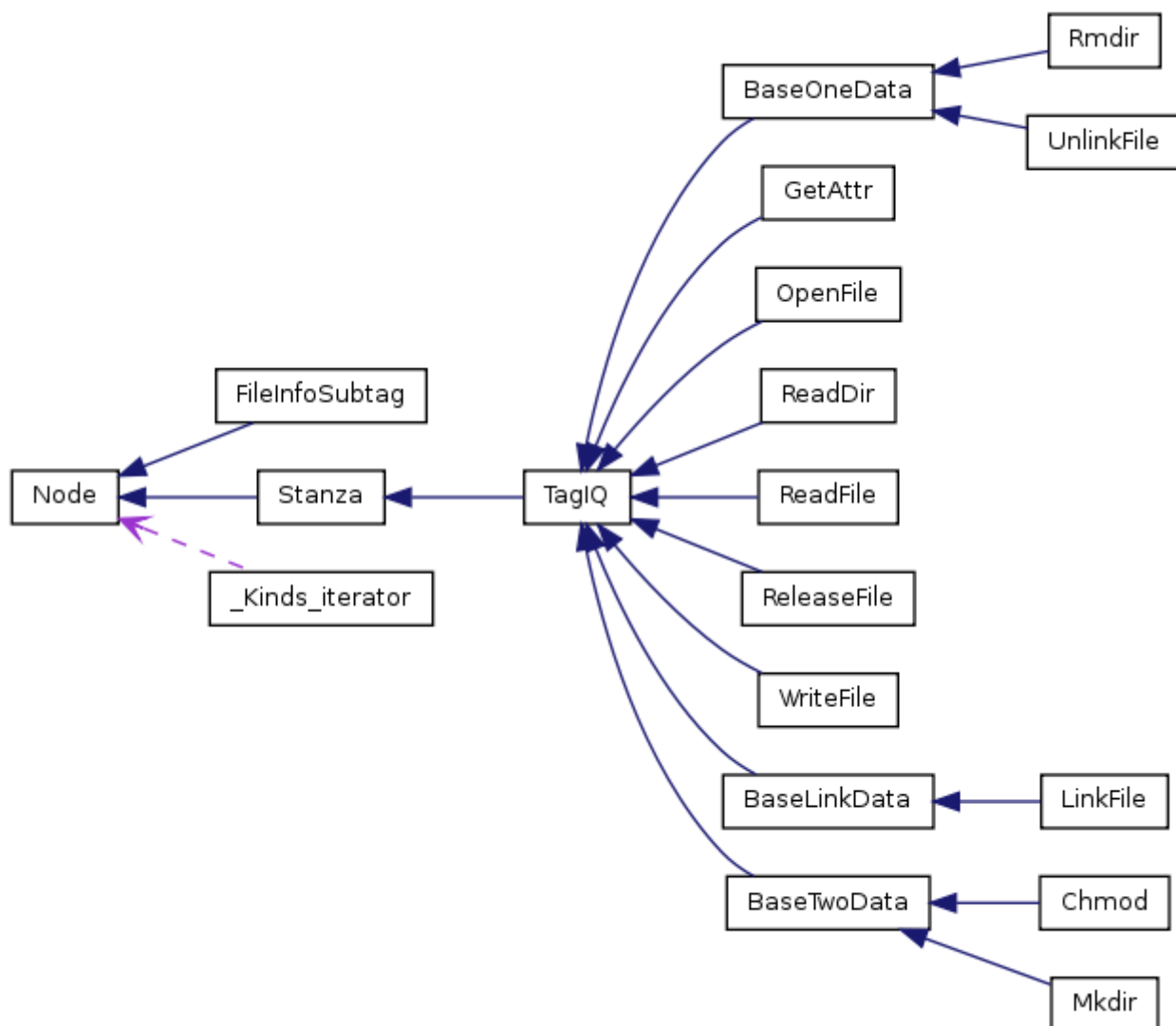
Рисунок 3.1 – Схема наследования классов реализующих построение XML
