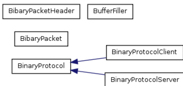
Рисунок 3.4 – Схема наследования классов бинарного протокола.
