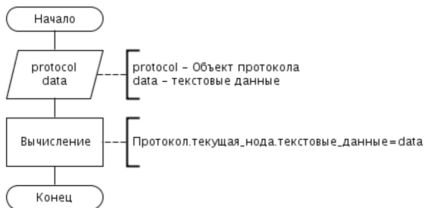
Рисунок 2.10 – Алгоритм обработки текстовых данных внутри тега принимает объект протокола на основе XML, из него извлекаются обработчики станз, а так-же текущая нода. Алгоритм выбирает первый обработчик, сравнивает подходит ли он для данной станзы, т.е. совпадает ли имя тега, его пространство имен (атрибут xmlns, являющийся уникальным для каждого типа
