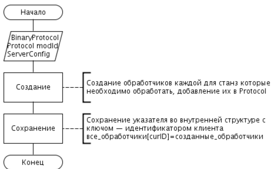
Рисунок 2.5 – Алгоритм регистрации модулей сервера
