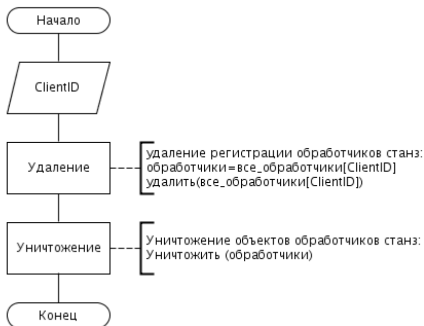
Рисунок 2.6 – Алгоритм удаления модулей сервера
