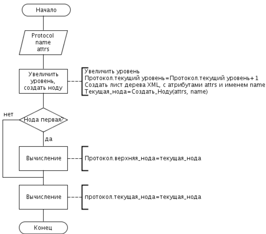
Рисунок 2.9 – Алгоритм обработки начала тега
