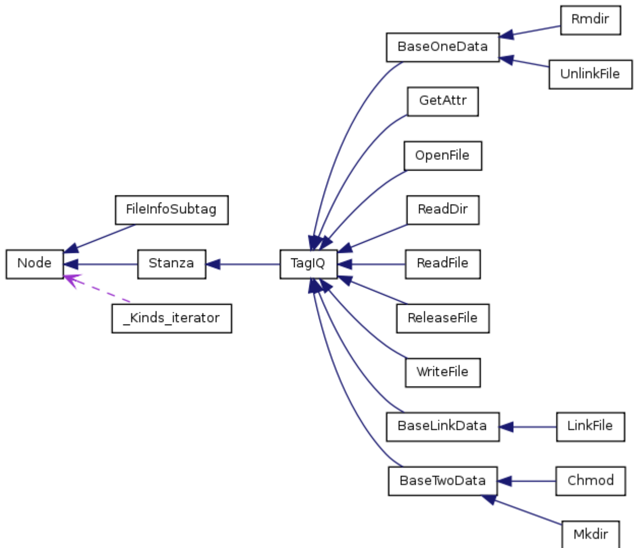
Рисунок 3.3 – Схема наследования классов реализующих построение XML
