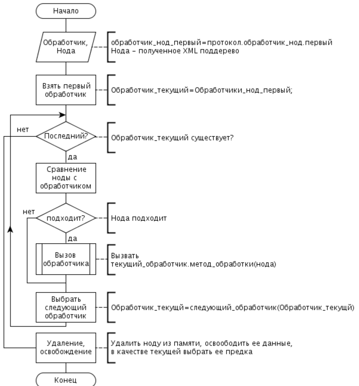
Рисунок 2.11 – Алгоритм обработки конца тега
