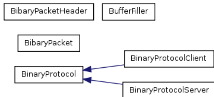
Рисунок 3.6 – Классы и структуры данных бинарного протокола
