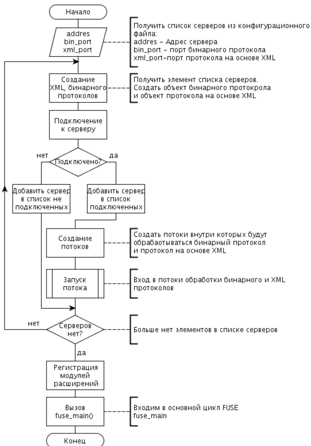
Рисунок 2.7 – Алгоритм подключения клиента к серверам
