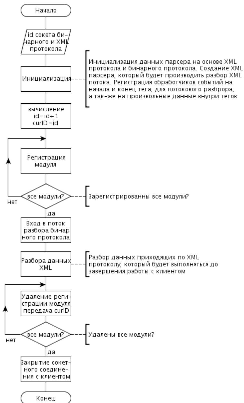
Рисунок 2.4 – Алгоритм цикла обработки клиента основе XML, указатель на объект бинарного протокола, указатель на конфигурационный файл сервера, и идентификатор регистрируемых модулей.
