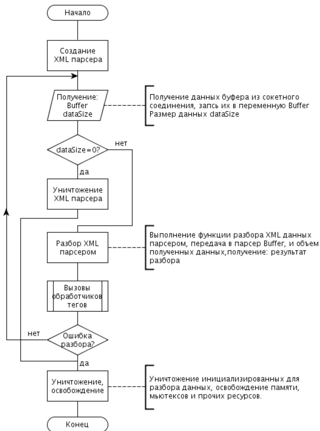
Рисунок 2.8 – Алгоритм разбора потокового XML
