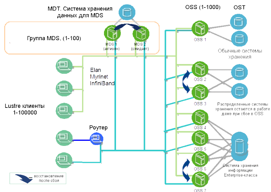
Рисунок 1.1 – Схема архитектуры системы Lustre
