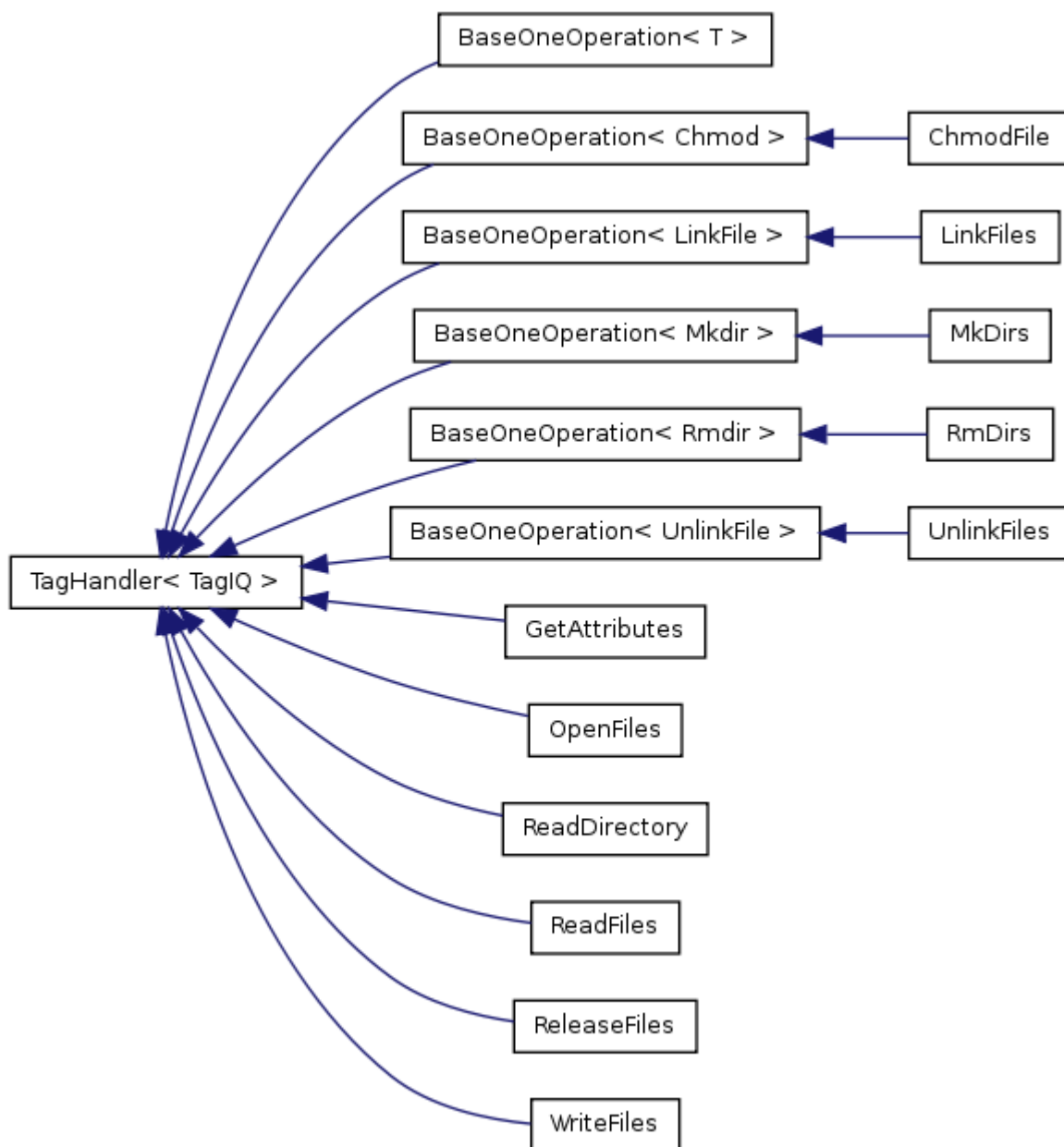
Рисунок 3.4 – Схема наследования классов обработки IQ запросов
