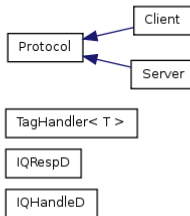
Рисунок 3.5 – Классы и структуры данных протокола на основе XML
